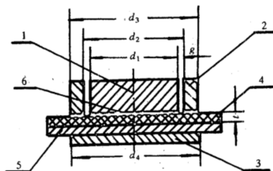
图 B.3.3 试件与电极配置
