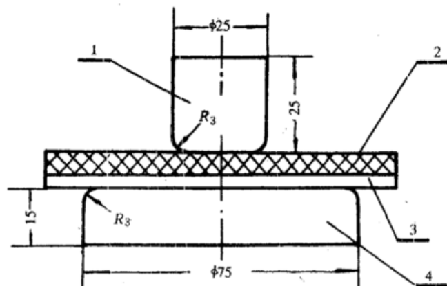
图 A.3.2 试件与电极配置
